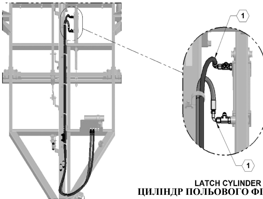
TOP VIEW ВИГЛЯД ЗВЕРХУ
